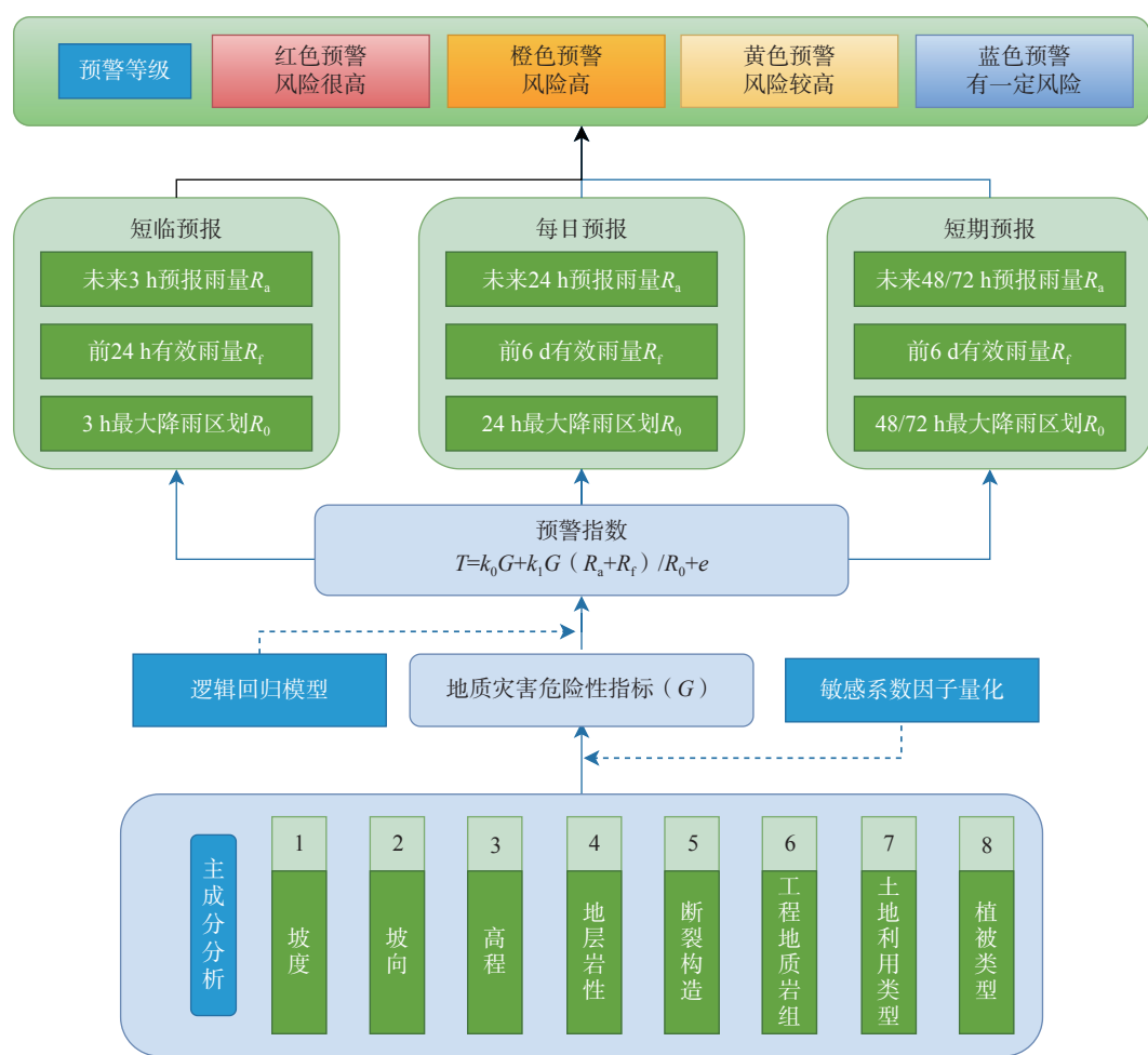
图 4 地质灾害气象风险预警模型方法
