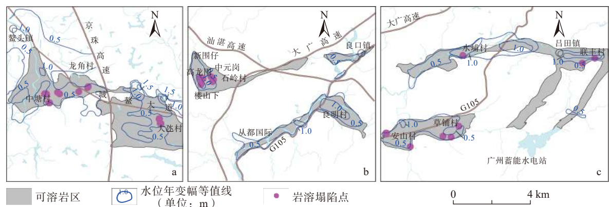
图 6 地下水水位年变幅分区图 Fig. 6 Zone map of annual variation of groundwater level
