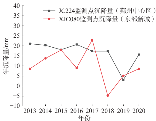
图 2 宁波市地面沉降速率图
