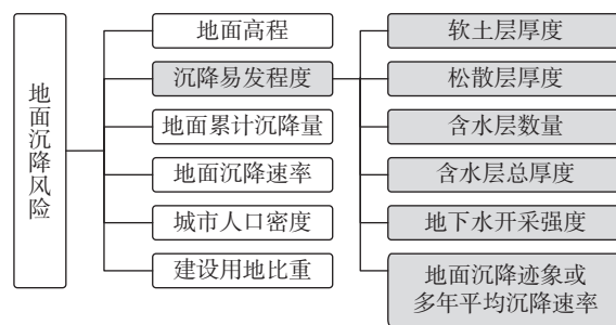
图 3 宁波市地面沉降风险评价体系
