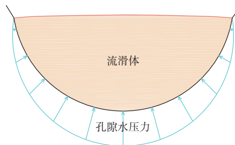
图 15 沟道中滑带孔隙水压力作用模式图
