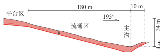
图 9 流通区滑速计算剖面简图
