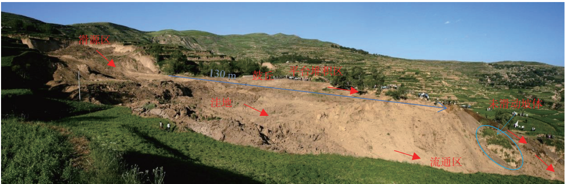
图 5 永光 1#滑坡滑源区—平台堆积区
