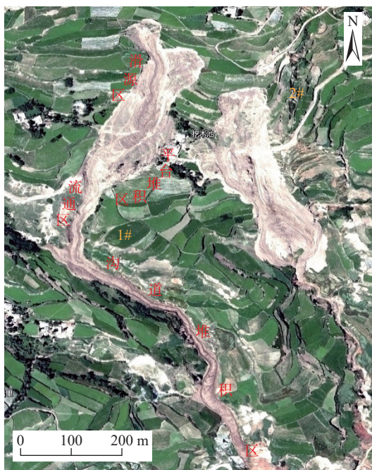
图 2 永光滑坡正射影像图
