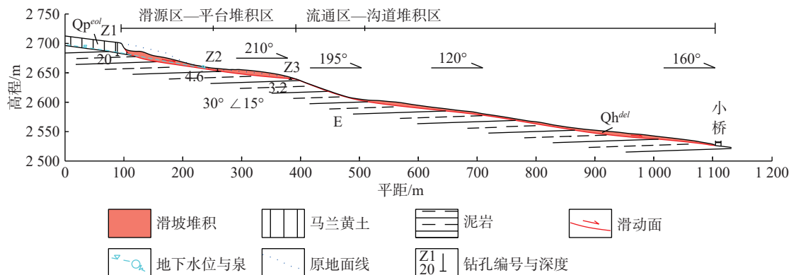
图 4 永光 1#滑坡工程地质剖面图
