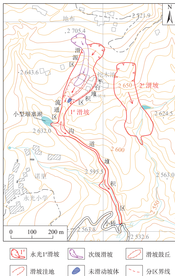
图 3 永光滑坡平面图
