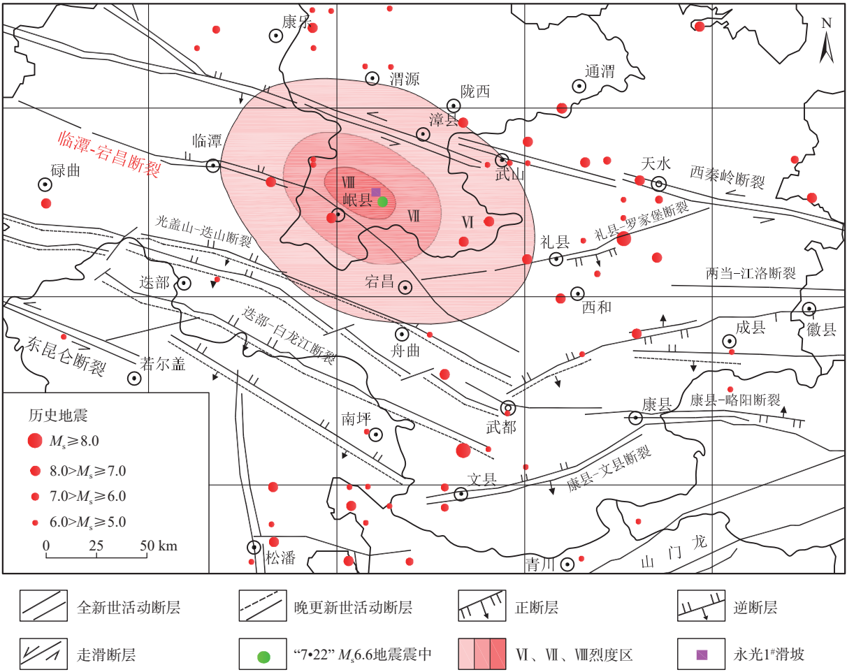
图 1 “7·22”岷县漳县地震烈度与构造背景图
