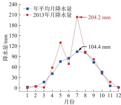
图 11 2013 年岷县降水量曲线 Fig. 11 The precipitation curve for Minxian County in 2013
