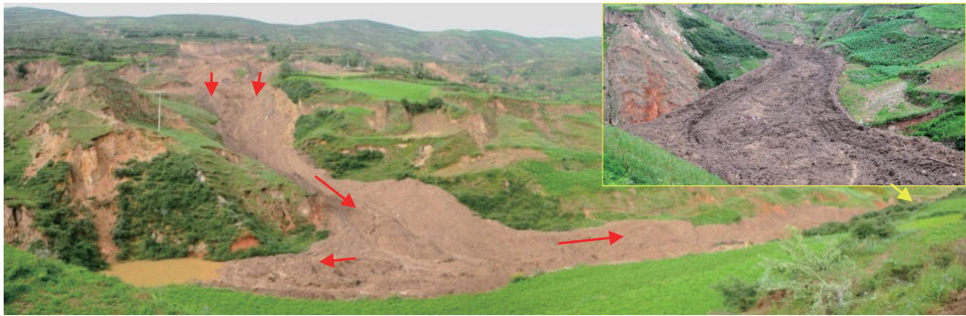
图 6 流通区—沟道堆积区及堰塞湖
