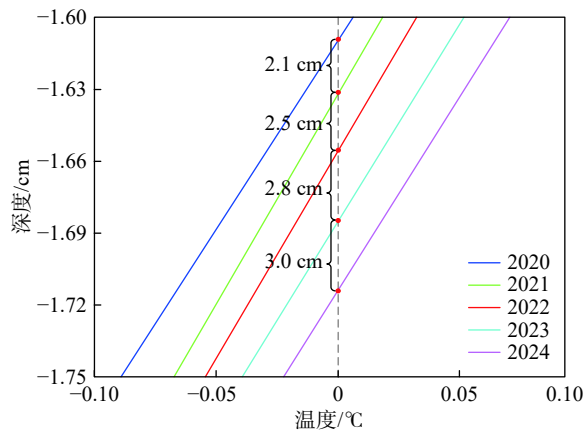
图 9 2020—2024 年 8 月 26 日 1-1' 测线地温随深度分布 Fig. 9 Depth distribution of ground temperature of 1-1' section on August 26 from 2020—2024
