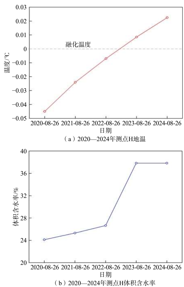
图 10 2020—2024 年测点 H 地温和体积含水率 Fig. 10 Ground temperature and volumetric water content of monitoring point H on 2020—2024
