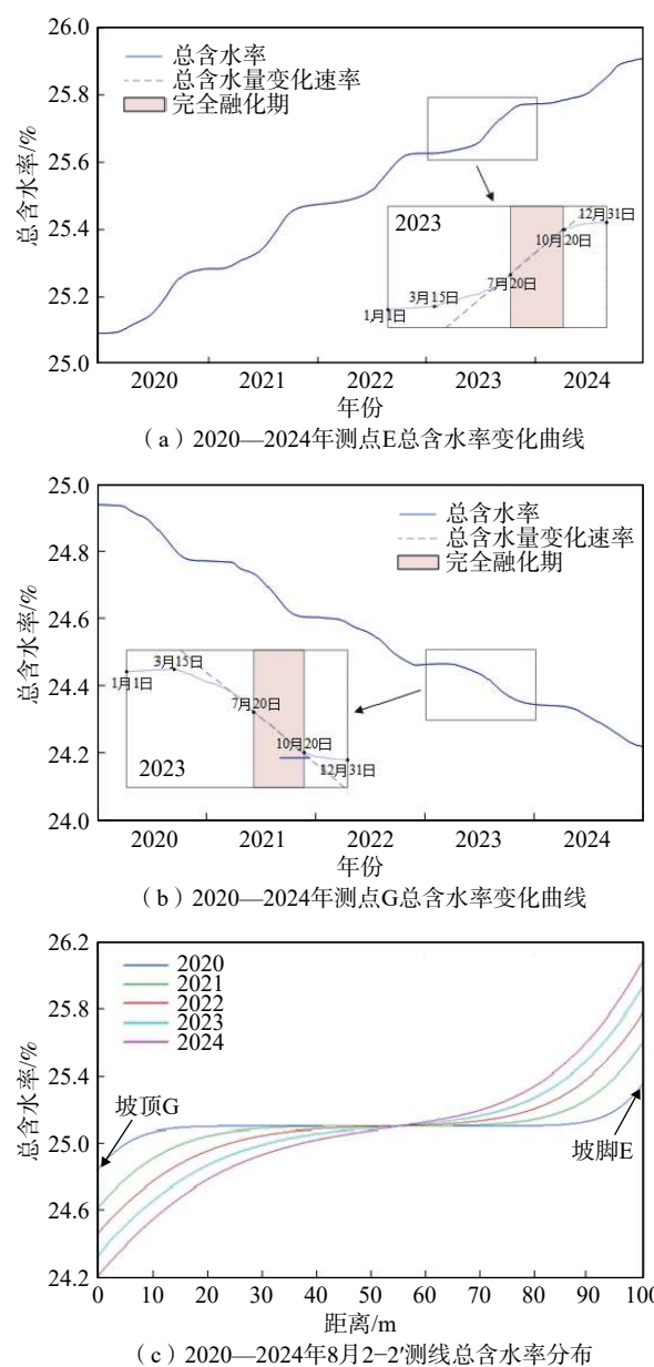
图 7 水分迁移规律 Fig. 7 Water migration rules
