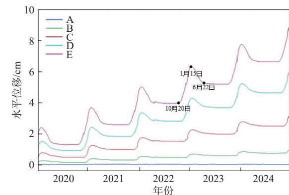
(a) 2020—2024年测线1-1'上测点A-E水平位移变化
