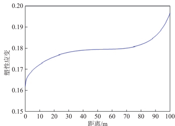
(b) 2024年12月测线2-2'塑性应变曲线
