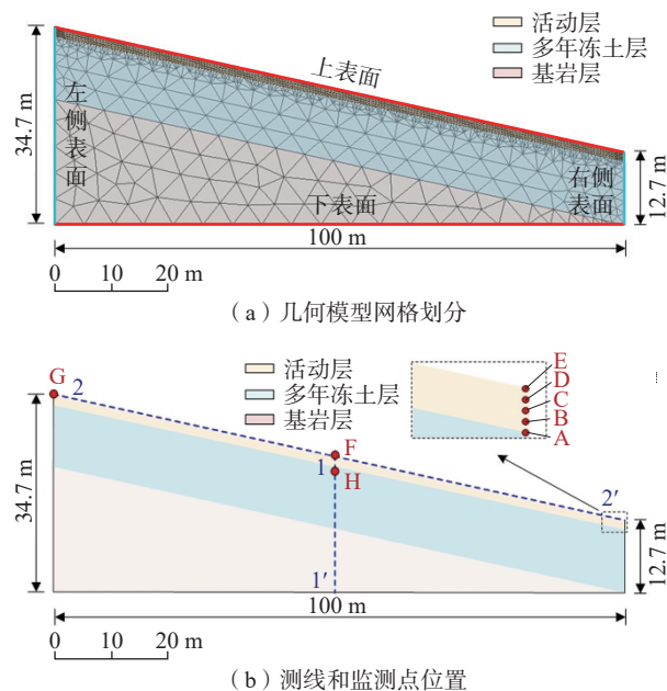
图 5 有限元计算模型 Fig. 5 Finite element computational model
