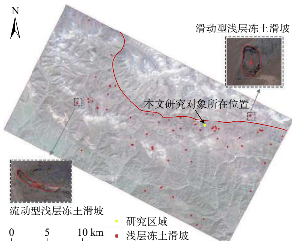
图 2 青海省祁连县重点工作区浅层冻土滑坡分布
