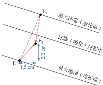
(c) 测点E冻胀融沉位移示意图
