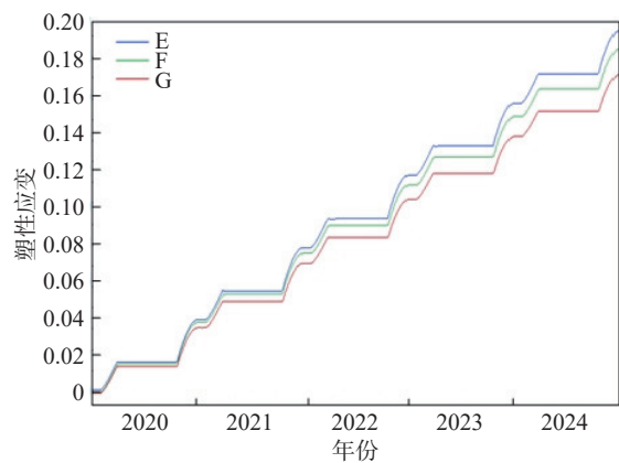
(a) 2020—2024年测线2-2'上测点E、F、G塑性应变变化曲线
