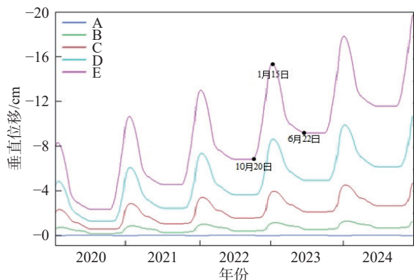
(b) 2020—2024年测线1-1'上测点A-E垂直位移变化
