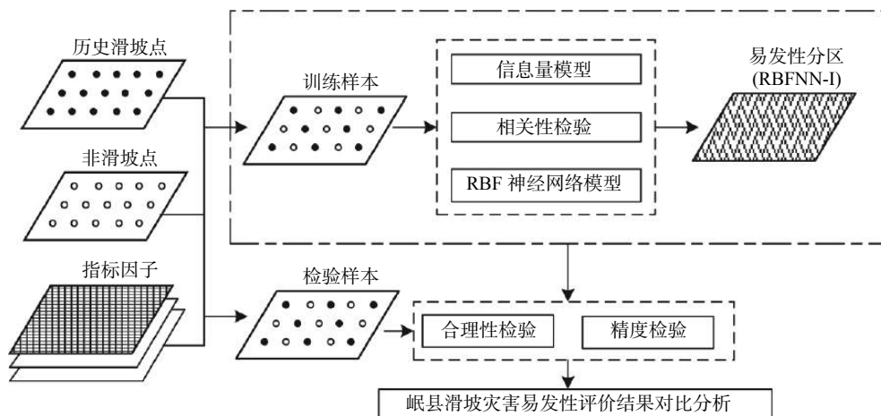
图 2 基于 RBFNN-I 模型滑坡灾害易发性评价流程图
